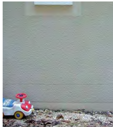
Figure 4 : La semelle a fléchi, insuffisamment soutenue par le sol. Une fissure s'ouvre entre le plancher et le soubassement.
