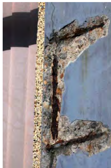
Figure 121 : Éclat de béton autour de l'armature d'un poteau insuffisamment enrobée.
