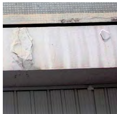
Figure 122 : Éclat de béton autour de l'armature d'un bandeau de façade. L'éclat se forme puis se détache.
